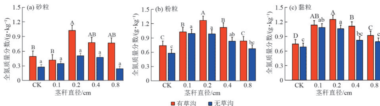
图4 不同茎秆直径下迁移泥沙中TN质量分数
